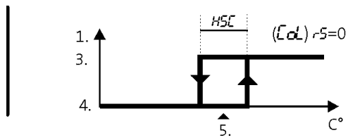
Heizbetrieb 2-Punkt
