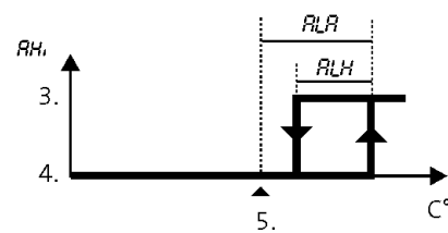
Alarm Übertemperatur
