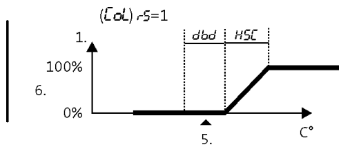
Heiz- und Kühlbetrieb P-Band
